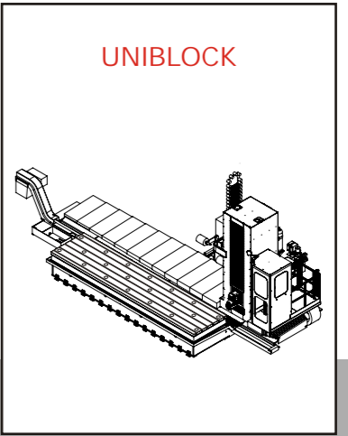
Montante, basamento e carro Column, bed and carriage Ständer, Bett und Karre Montant, bâti et char
