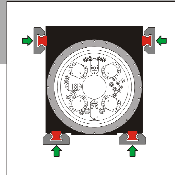
Asse trasversale - 8 pattini su 4 guide Cross axis - 8 runners on 4 guideways Quer Achse - 8 Rollschuhe auf 4 Führungen Axe transversal - 8 patins sur 4 glissières
