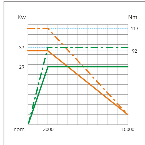
MOTORE AC SINCRONO • SYNCHRONOUS-MOTOR SYNCHRON-MOTOR • MOTEUR SYNCHRONE
